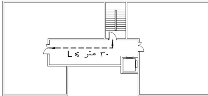
شکل ۴-۲-۵- فاصله درب واحد تا پلکان خروج در ساختمان فاقد شبکه بارنده خودکار
