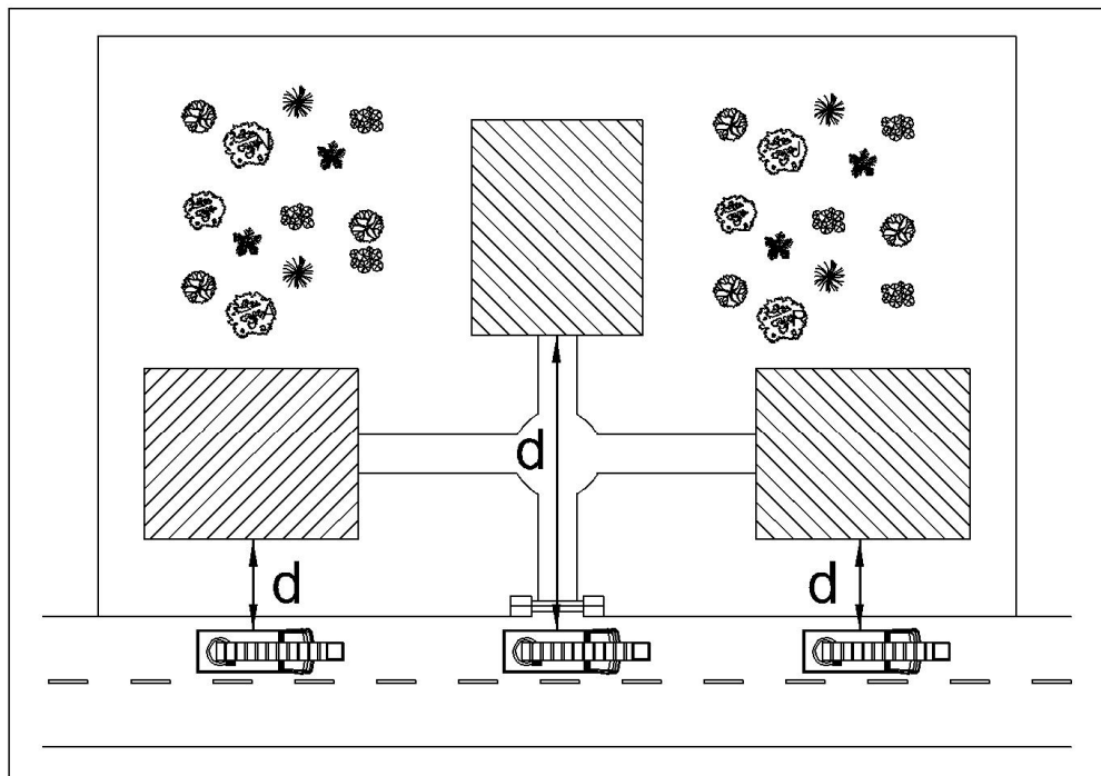
شکل ۳-۲-۵-الف- استقرار خودروی امدادی داخل مجتمع
