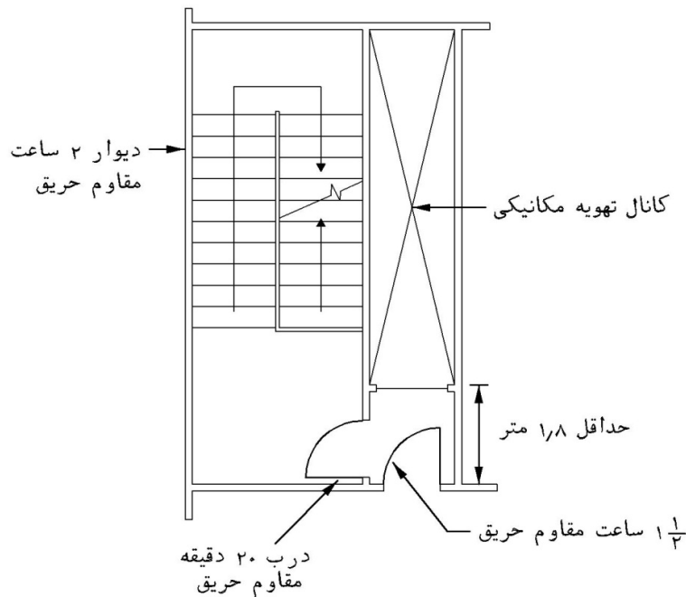
شکل ۴-۳-۴- استفاده از پیش ورودی با تهویه مکانیکی
