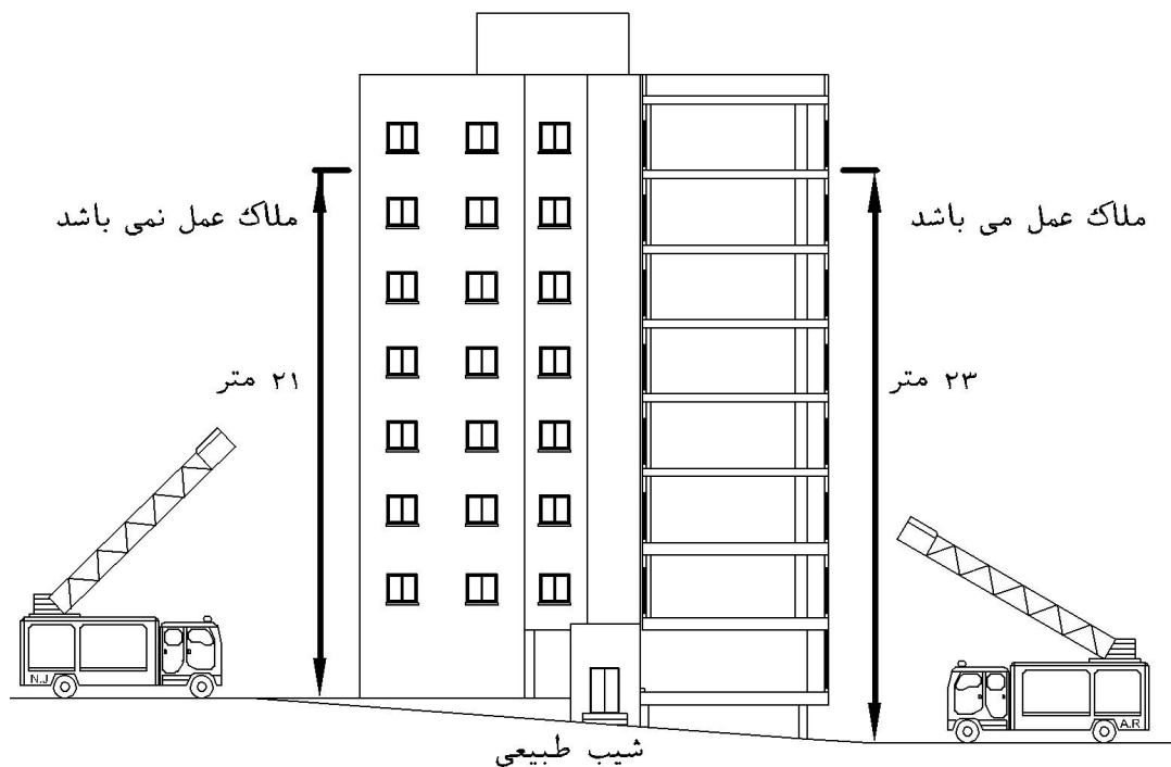
شکل ۵-۱-۲- نحوه اندازه گیری ارتفاع
