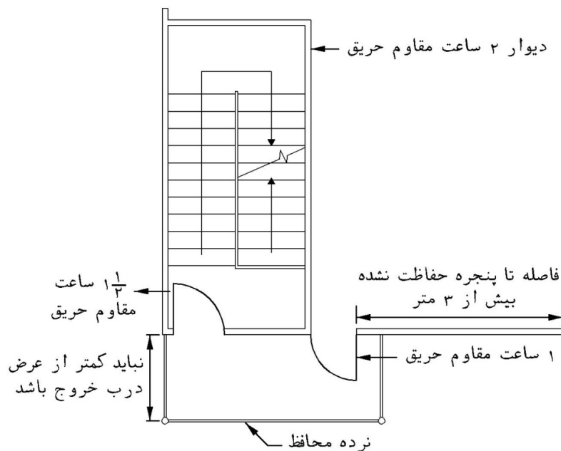
شکل ۲-۴-۴- استفاده از بالکن با تهویه طبیعی
