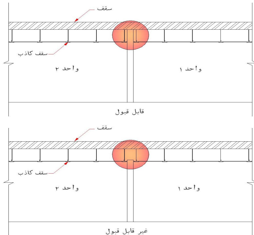
شکل ۵-۶-۲- ارتباط بین واحدها از طریق سقف کاذب
