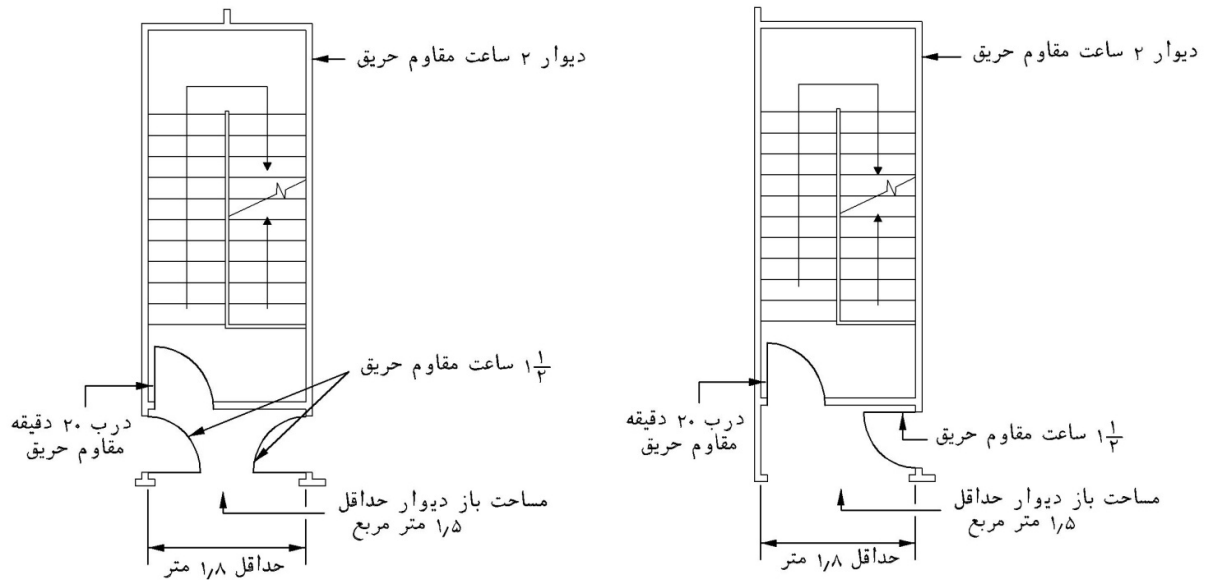
شکل ۱-۴-۴- استفاده از پیش ورودی با تهویه طبیعی
