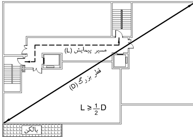
شکل شماره ۲-۲-۴- نحوه محاسبه فاصله بین دو پله
