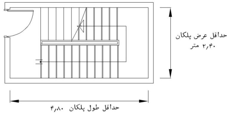
شکل ۳-۳-۴- ابعاد پلکان
