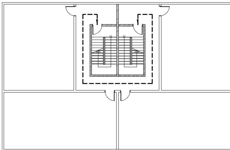
شکل ۴-۱-۷- پلکان‌های به هم چسبیده
